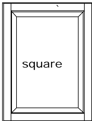
W-1 1 PANEL MIN. 7"W X 7"H
