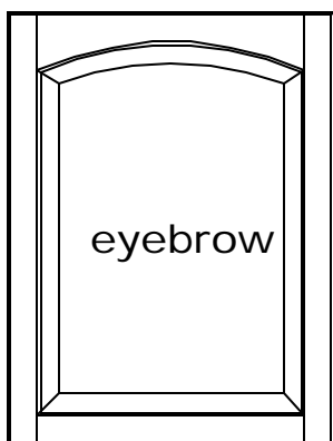
W-2 1 PANEL MIN. 8 1/2"W X 9"H
