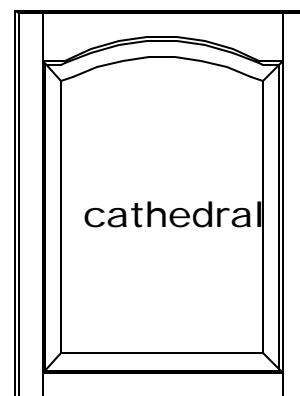
W-3 1 PANEL MIN. 9 1/2"W X 9"H
